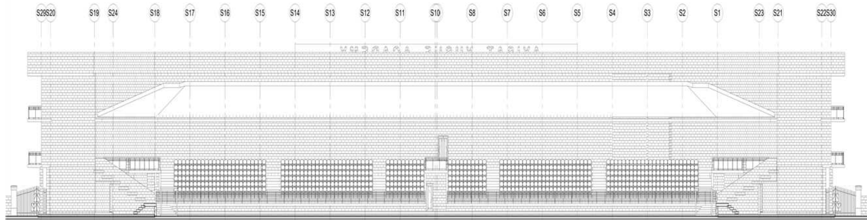
SECTION A-A
